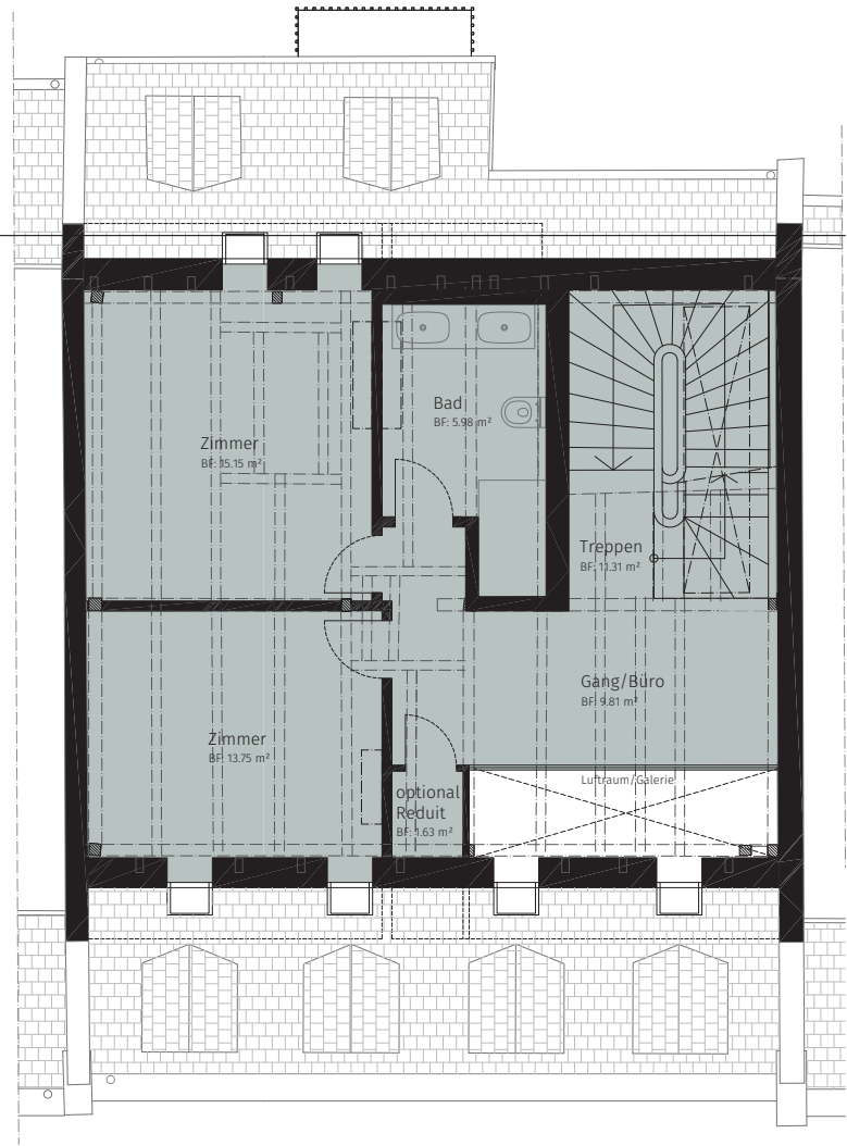
2. Dachgeschoss
